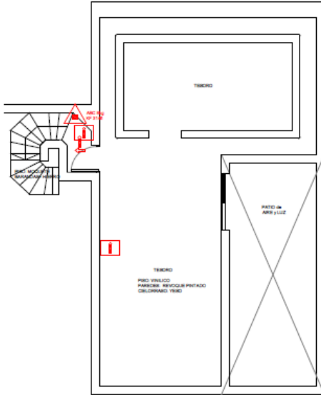
PLANTA SUBSUELO
