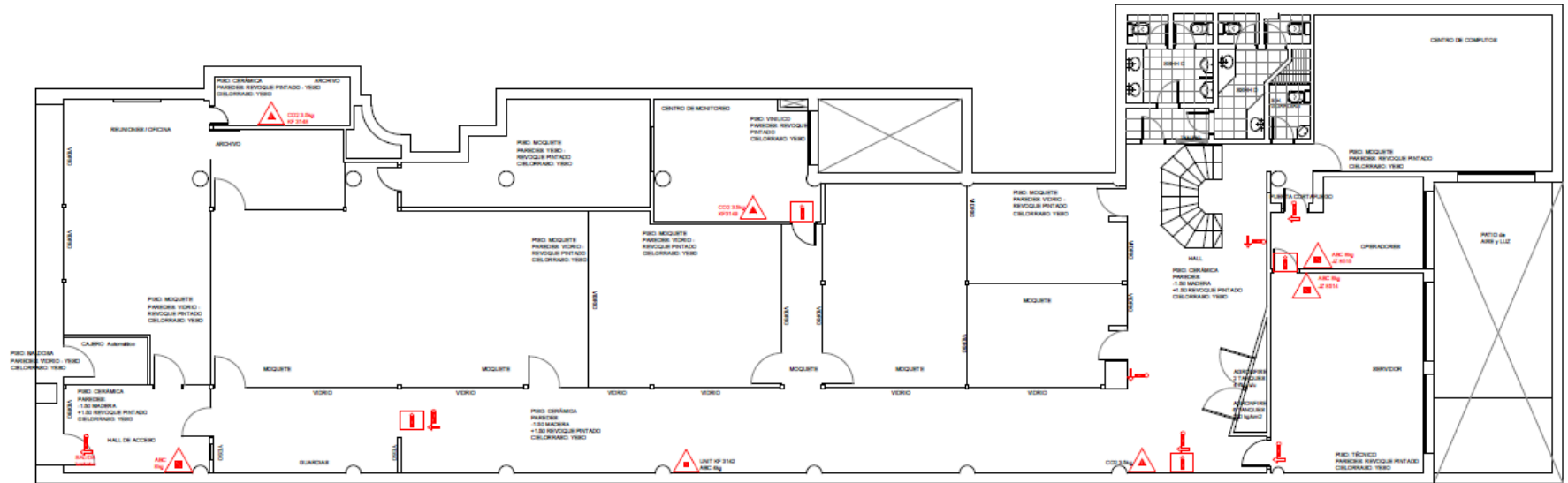
PLANTA BAJA
