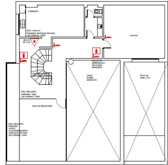
PLANTA ENTREPISO
