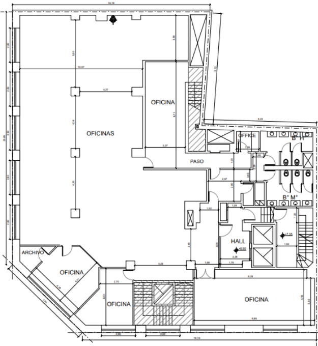
Piso 2°
