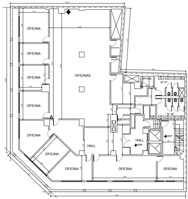
Piso 6°
